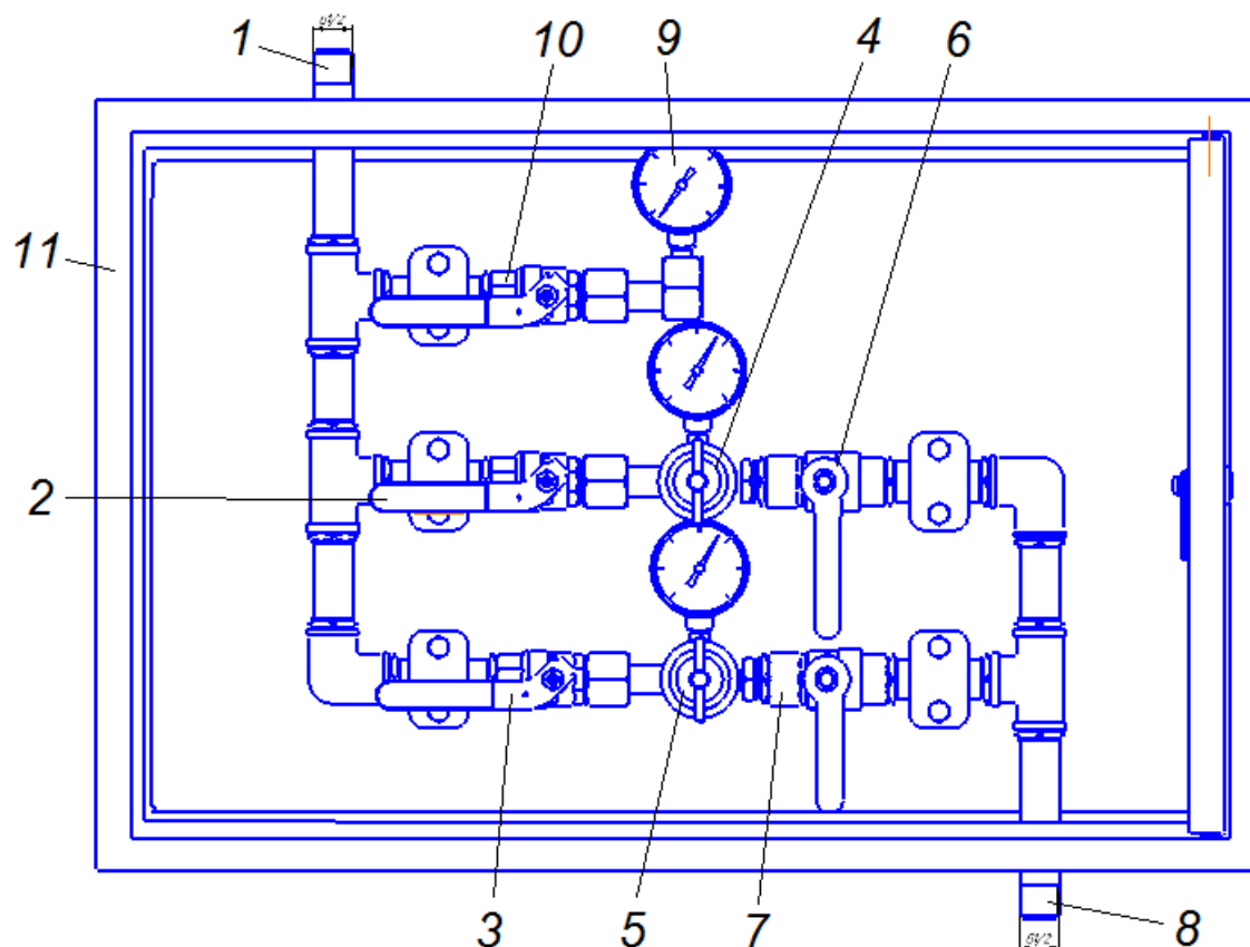
Рис.1 Пост газоразборный: а - ПГК-10x2-з
